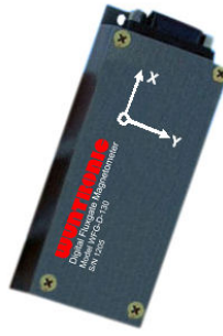
3-achsiges Fluxgate Magnetometer mit Digitalausgang.
